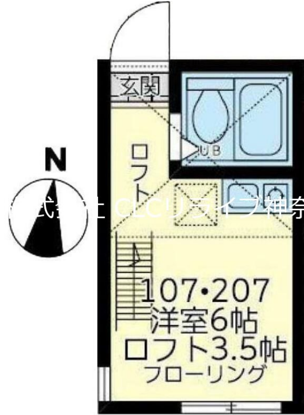
【間取り図】
