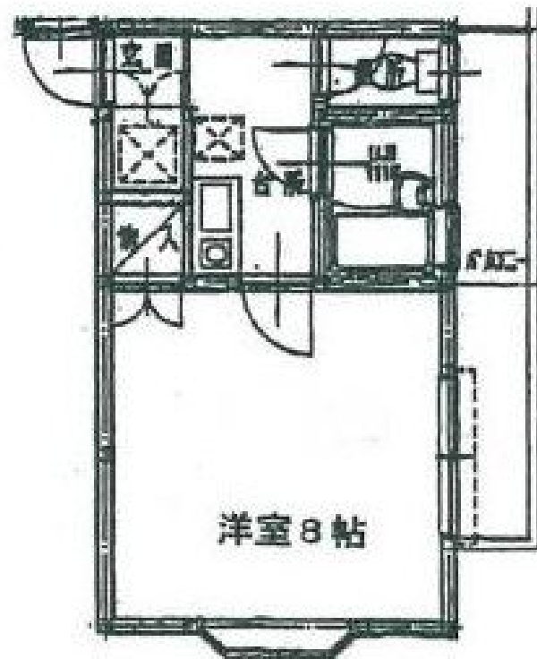
【間取り図】
